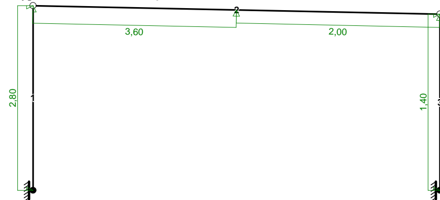
Przypadek P5 : wiatr z prawej ( \square_f = 1,5 )
